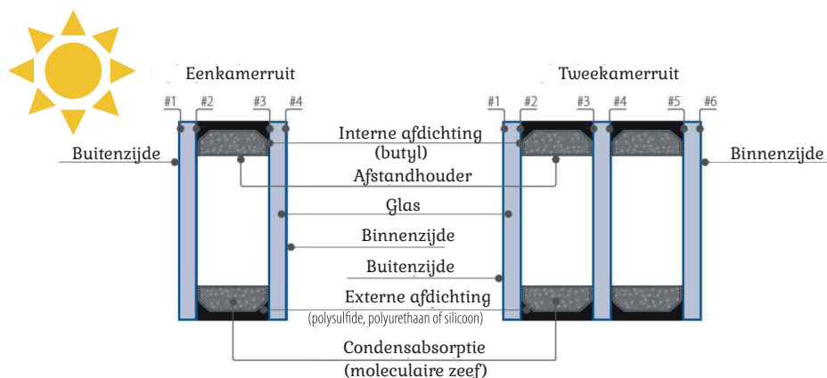
Afb. 1 Opbouw van een eenkamer- en tweekamerruit met markering van de onderdelen
